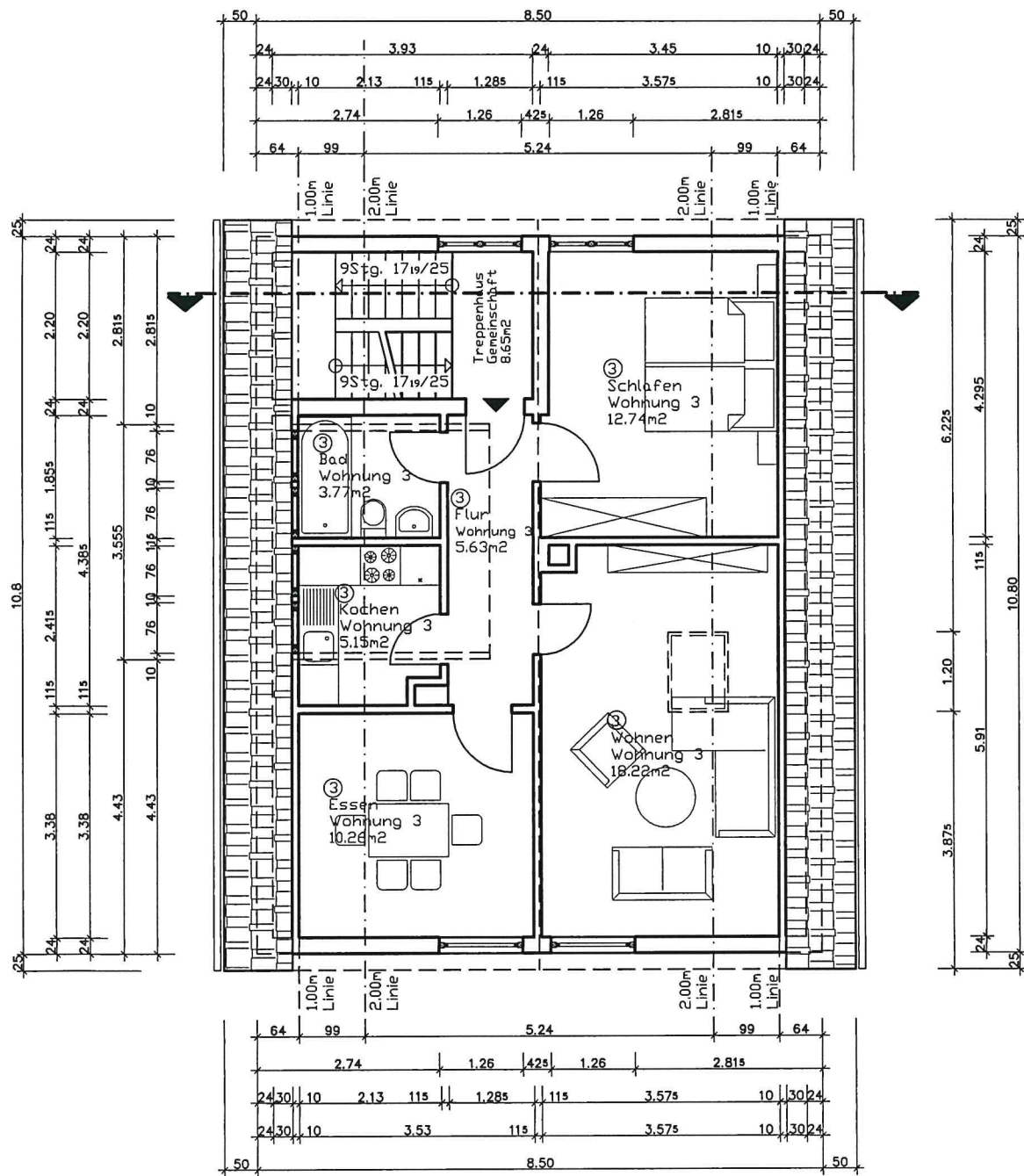
Dachgeschoss
