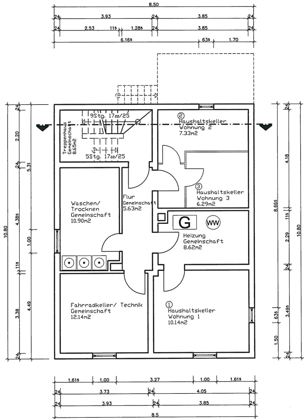
Kellergeschoss
