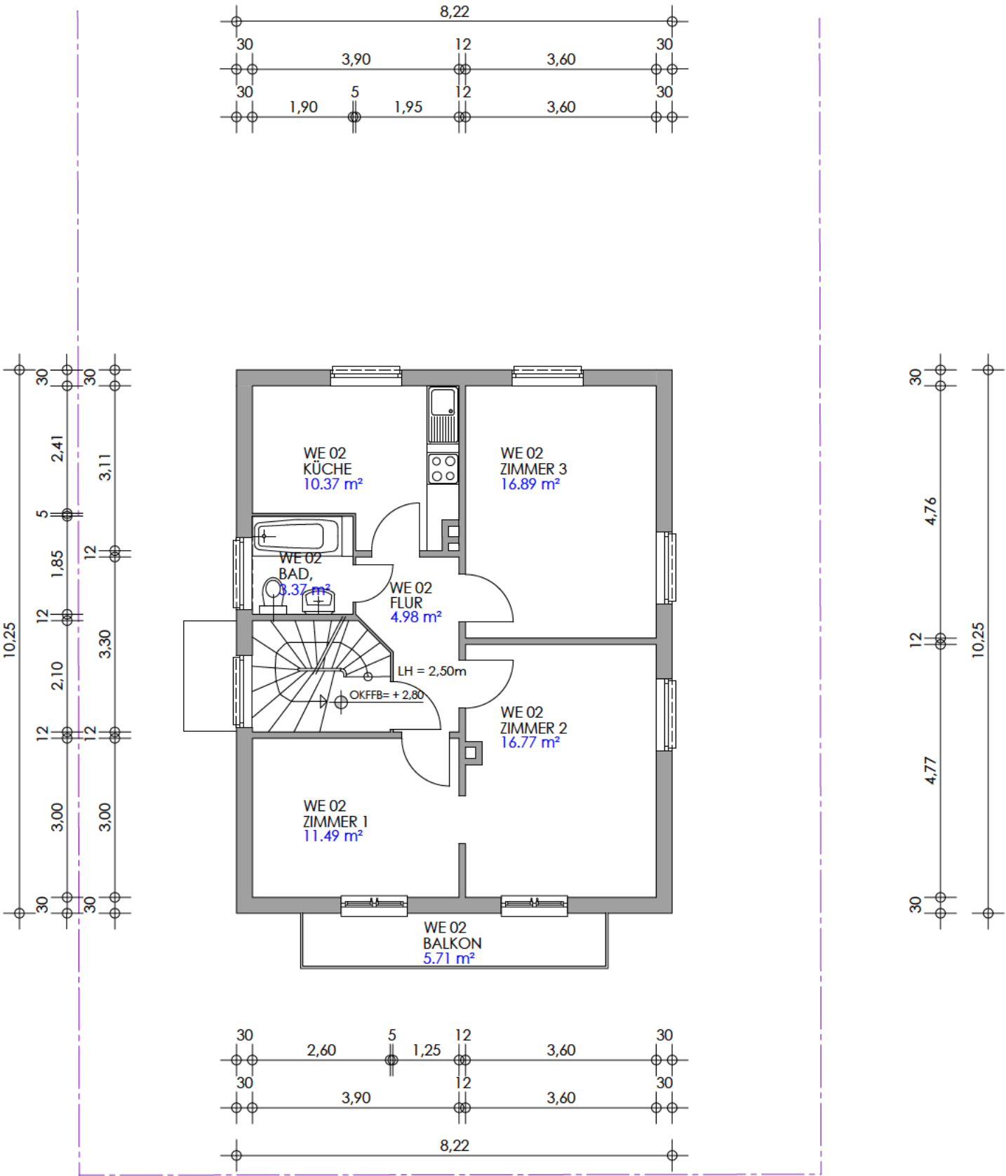
OBERGESCHOSS
